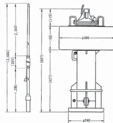
●外観寸法図(単位/mm)
